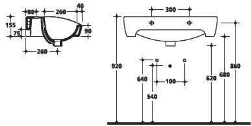
3341 Lavabo 75x45 incasso o sospeso monoforo One hole wall hung or inset basin 75x45
