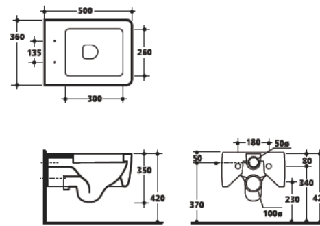
3215 Vaso sospeso Wall hung wc
