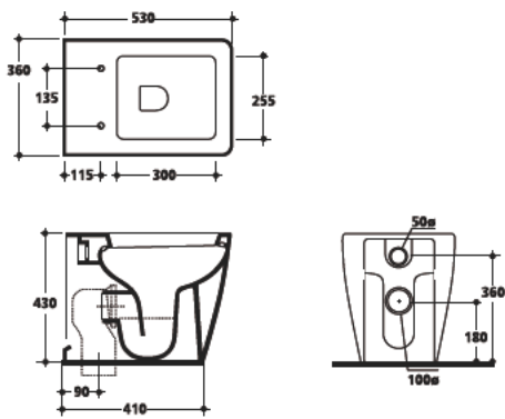
3216 Vaso unico 53 cm scarico a parete "P" completo di curva tecnica per scarico suolo "S" Btw wc pan 53 cm wall outlet with waste pipe floor outlet
