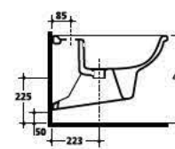
2325 Bidet sospeso monoforo One hole wall hung bidet
