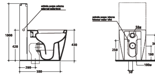
3216 Vaso unico 53 cm scarico a parete "P" completo di curva tecnica per scarico suolo "S" Btw wc pan 53 cm wall outlet with waste pipe floor outlet
