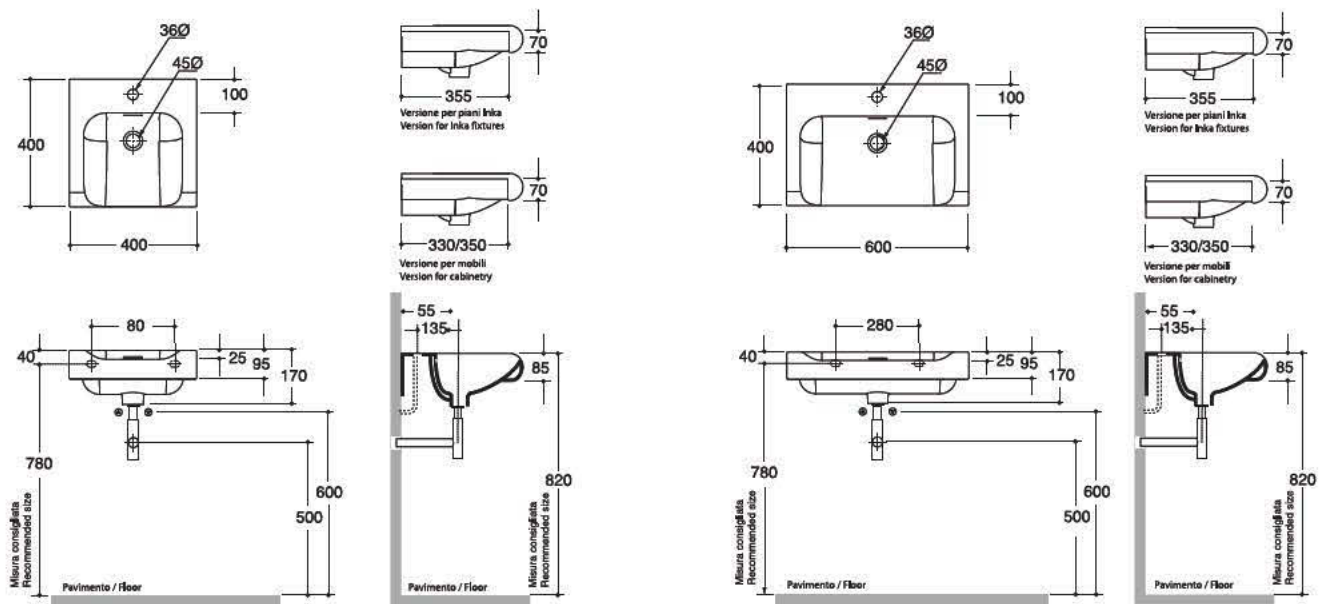
3412 Lavabo semincasso 40x40x35,5 monoforo One hole semi recessed washbasin 40x40x35,5
