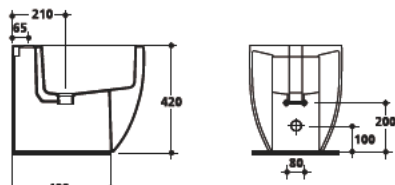
3120 Bidet monoforo 52 cm One hole bidet 52 cm
