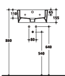
3149 Lavabo 40x37 cm sospeso o appoggio monoforo One hole wall hung or free standing washbasin 40x37 cm
