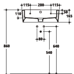
3141 Lavabo 50x40 cm sospeso o appoggio monoforo One hole wall hung or free standing washbasin 50x40 cm
