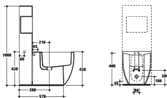
3120 Bidet monoforo 52 cm One hole bidet 52 cm
