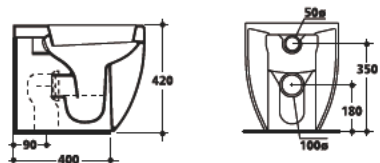
3116 Vaso unico 52 cm scarico a parete "P" completo di curva tecnica per scarico suolo "S" Btw wc pan 52 cm wall outlet with waste pipe floor outlet
