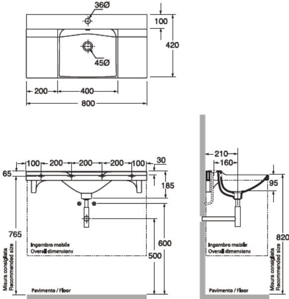
3403 BUDDY Lavabo 80x42 appoggio o sospeso monoforo BUDDY One hole wall hung or free standing washbasin 80x42
