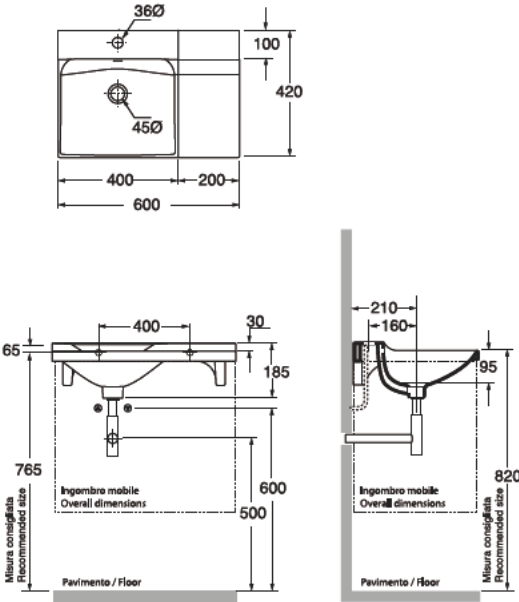
3402 BUDDY Lavabo 60x42 appoggio o sospeso monoforo BUDDY One hole wall hung or free standing washbasin 60x42
