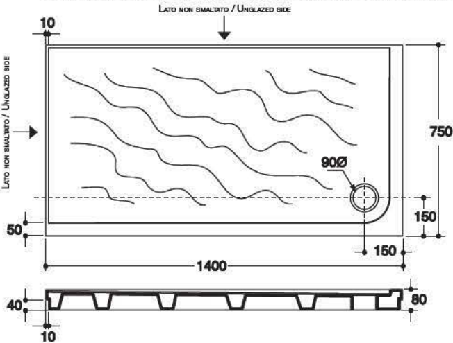
SABBIA Piatto doccia angolare SX 140x75xh4 rectangular shaped "Sabbia" corner shower tray 140x75xh4 left side
