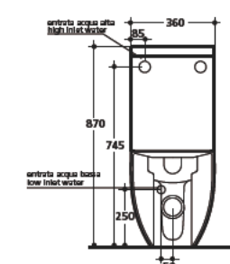
3117 Vaso monoblocco unico scarico a parete "P" completo di curva tecnica per scarico suolo "S" Close coupled wc pan wall outlet with waste pipe floor outlet
