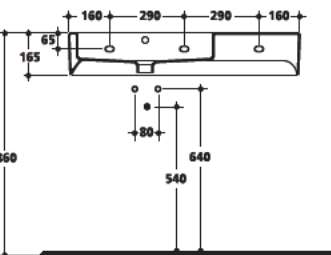
3144 Lavabo 90x42 cm sospeso o appoggio monoforo vasca asimmetrica One hole wall hung or freestanding asymmetrical washbasin 90x42 cm
