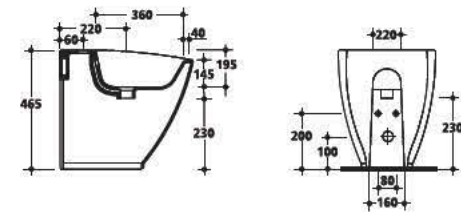
3320 Bidet monoforo One hole bidet
