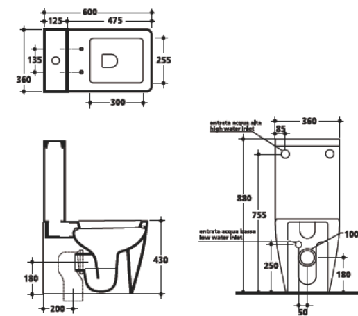
3217 Vaso monoblocco unico scarico a parete "P" completo di curva tecnica per scarico suolo "S" Close coupled wc pan wall outlet with waste pipe floor outlet
