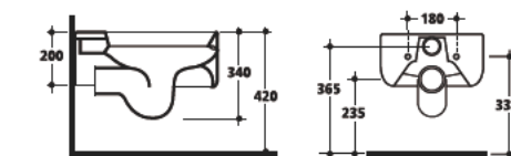
3115 Vaso sospeso Wall hung wc
