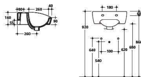
3340 Lavabo 45x45 incasso o sospeso monoforo One hole wall hung or inset basin 45x45
