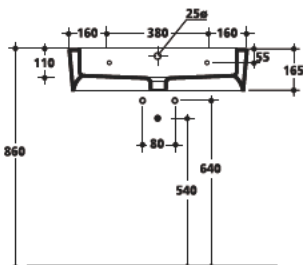
3250 Lavabo 70x43 cm sospeso o appoggio monoforo One hole wall hung or free standing washbasin 70x43 cm
