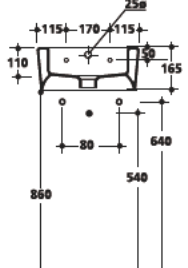
3249 Lavabo 40x40 cm sospeso o appoggio monoforo One hole wall hung or free standing washbasin 40x40 cm
