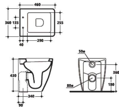
3214 Vaso unico 46 cm. scarico a parete "P" completo di curva tecnica per scarico suolo "S" Btw wc pan 46 cm. wall outlet with waste pipe floor outlet
