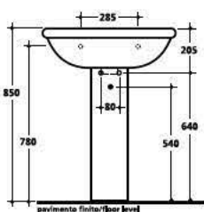
2366 - 2370 Lavabo 66 cm su colonna Washbasin 66 cm on pedestal
