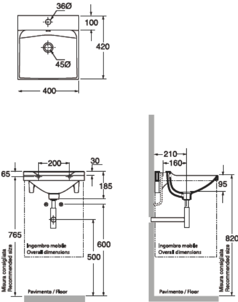
3401 BUDDY Lavabo 40x42 appoggio o sospeso monoforo BUDDY One hole wall hung or free standing washbasin 40x42
