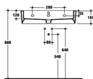
3150 Lavabo 70x42 cm sospeso o appoggio monoforo One hole wall hung or free standing washbasin 70x42 cm
