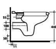
2315 Vaso sospeso Wall hung wc pan
