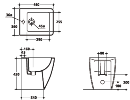
3221 Bidet monoforo 46 cm. One hole bidet 46 cm.
