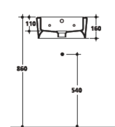
3147 Lavabo 40x32 cm sospeso o appoggio Wall hung or free standing washbasin 40x32 cm
