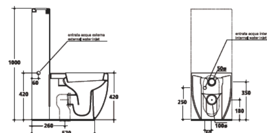
3116 Vaso unico 52 cm scarico a parete "P" completo di curva tecnica per scarico suolo "S" Btw wc pan 52 cm wall outlet with waste pipe floor outlet
