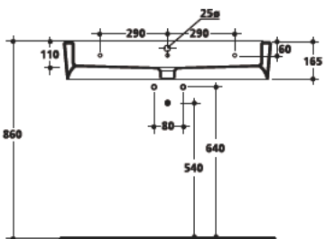
3251 Lavabo 90x43 cm sospeso o appoggio monoforo One hole wall hung or free standing washbasin 90x43 cm
