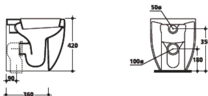
3114 Vaso unico 48 cm scarico a parete "P" completo di curva tecnica per scarico suolo "S" Btw wc pan 48 cm wall outlet with waste pipe floor outlet
