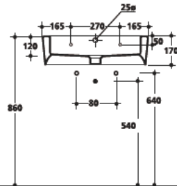
3242 Lavabo 60x43 cm sospeso o appoggio monoforo One hole wall hung or free standing washbasin 60x43 cm
