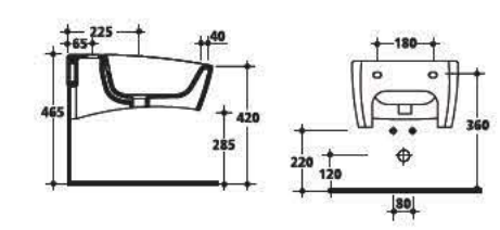
3325 Bidet sospeso monoforo One hole wall hung bidet
