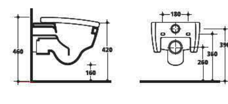
3315 Vaso sospeso Wall hung wc
