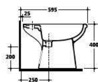
2320 Bidet monoforo One hole bidet
