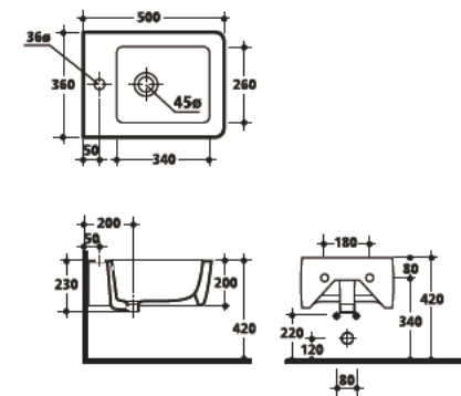
3225 Bidet sospeso monoforo One hole wall hung bidet
