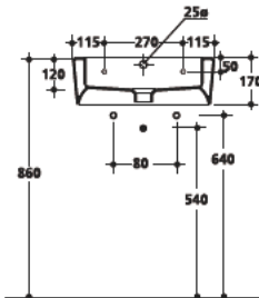
3241 Lavabo 50x40 cm sospeso o appoggio monoforo One hole wall hung or free standing washbasin 50x40 cm
