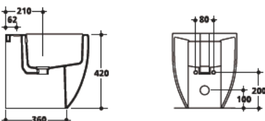
3121 Bidet monoforo 48 cm One hole bidet 48 cm
