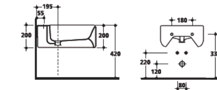
3125 Bidet sospeso monoforo One hole wall hung bidet
