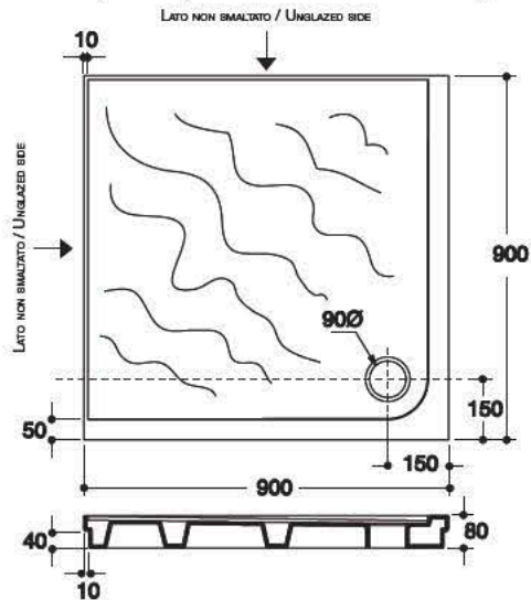
SABBIA Piatto doccia angolare 90x90xh4 square shaped "Sabbia" corner shower tray 90x90xh4
