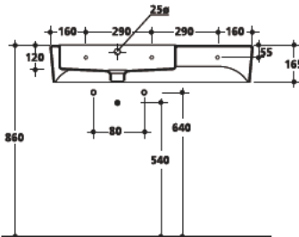
3244 Lavabo 90x43 cm sospeso o appoggio monoforo vasca asimmetrica One hole wall hung or freestanding asymmetrical washbasin 90x43 cm
