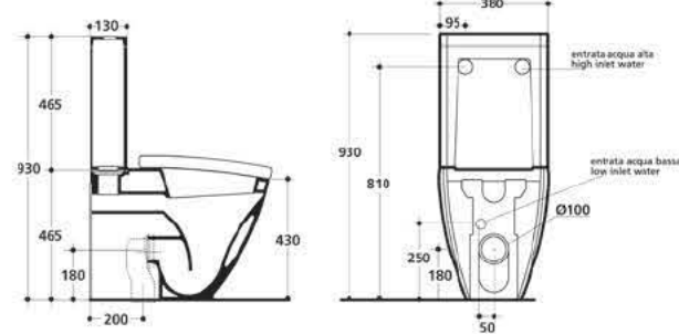
3317 Vaso monoblocco unico scarico a parete "P" completo di curva tecnica per scarico suolo "S" Close coupled wc pan wall outlet with waste pipe floor outlet
