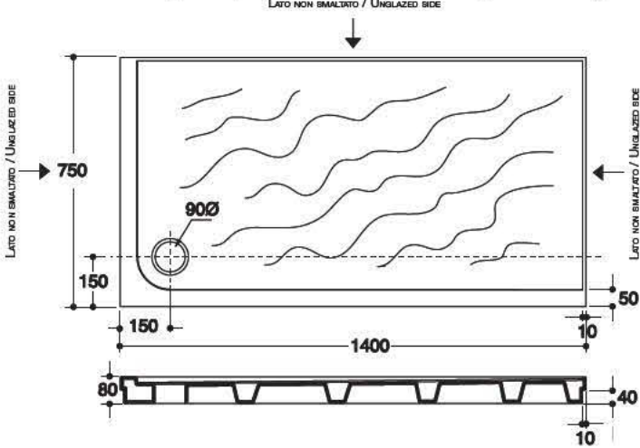
SABBIA Piatto doccia angolare DX 140x75xh4 rectangular shaped "Sabbia" corner shower tray 140x75xh4 right side
