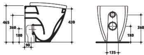
3316 Vaso unico scarico a parete "P" completo di curva tecnica per scarico suolo "S" Btw wc pan wall outlet with waste pipe floor outlet
