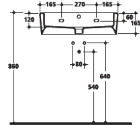
3142 Lavabo 60x42 cm sospeso o appoggio monoforo One hole wall hung or free standing washbasin 60x42 cm
