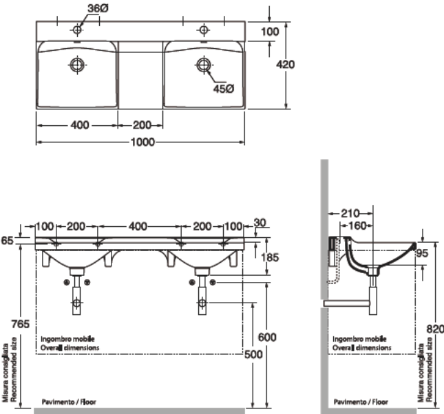
3404 BUDDY Lavabo 100x42 doppia vasca, appoggio o sospeso monoforo BUDDY Wall hung or free standing washbasin 100x42 double basin
