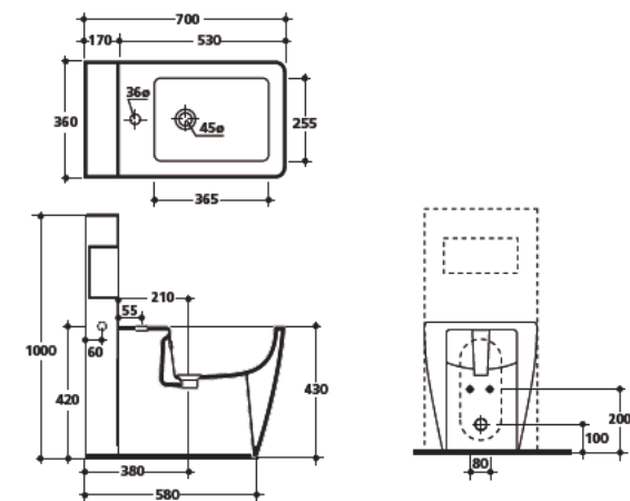
3220 Bidet monoforo 53 cm One hole bidet 53 cm
