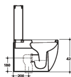
3117 Vaso monoblocco unico scarico a parete "P" completo di curva tecnica per scarico suolo "S" Close coupled wc pan wall outlet with waste pipe floor outlet
