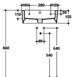
3140 Lavabo 46x37 cm sospeso o appoggio monoforo One hole wall hung or free standing washbasin 46x37 cm
