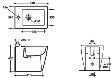
3220 Bidet monoforo 53 cm One hole bidet 53 cm
