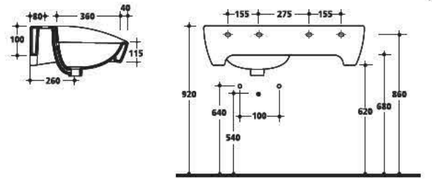
3343 Lavabo 90x55 sospeso monoforo One hole wall hung washbasin 90x55
