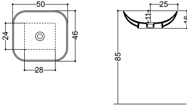
ART. 15081 lavabo da appoggio 50 senza piano rubinetteria overtop basin 50 without tap hole
