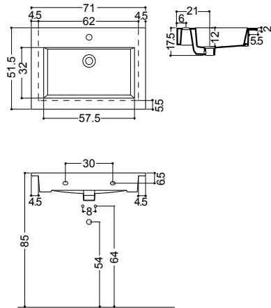
ART. WS330 consolle incasso 71 monoforo inset console 71 1/hole
