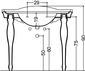
ART. 06039 lavabo incasso 68 monoforo/tre fori su richiesta inset basin 68 1/hole (3/holes upon request)
