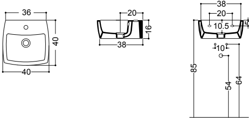
ART. 19090 lavabo da appoggio e sospeso 40 monoforo overtop or wall-hung basin 40 1/hole
