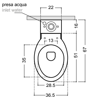
ART. 4417 vaso monoblocco monobloc wc
