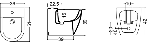
ART. 25022 bidet 51 monoforo BTW bidet 51 1/hole
