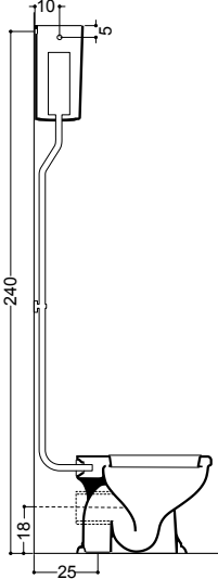
ART. 06010 vaso S. floor trap wc
