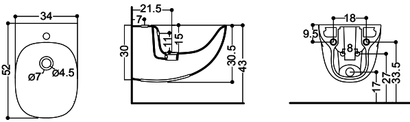
ART. 30022 bidet monoforo BTW bidet 1/hole
