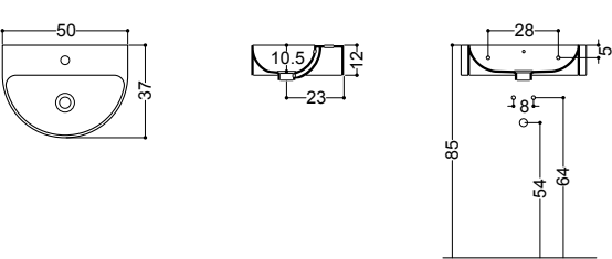
ART. WS118 lavabo da appoggio e sospeso 50 monoforo overtop or wall-hung basin 50 1/hole
