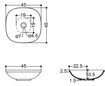
ART. 30090 lavabo incasso e soprapiano 45 senza piano rubinetteria semi inset basin 45 without tap hole
