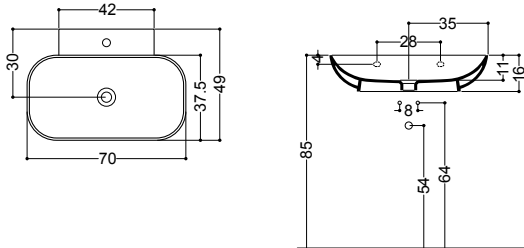
ART. 15092 lavabo appoggio e sospeso 70 monoforo overtop or wall-hung basin 70 1/hole
