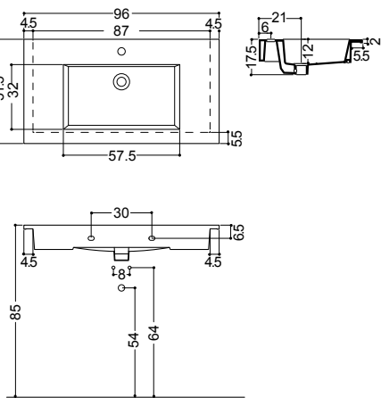
ART. WS324 consolle incasso 96 monoforo inset console 96 1/hole
