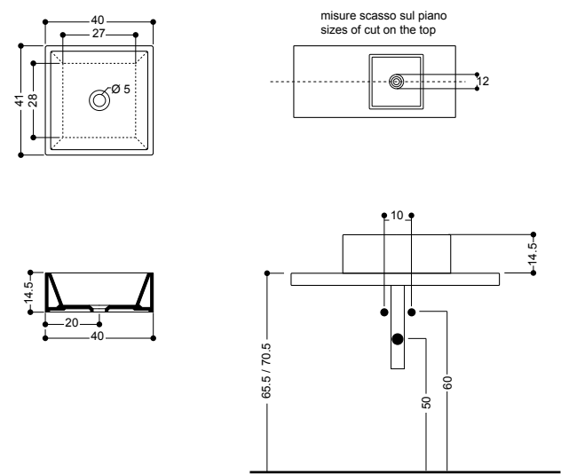
ART. WS019 lavabo da appoggio 40 senza piano rubinetteria overtop basin 40 without tap hole
