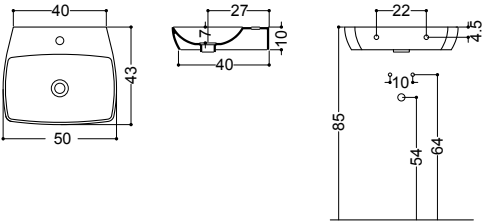
ART. 81091 lavabo da appoggio e sospeso 50 monoforo overtop or wall-hung basin 50 1/hole
