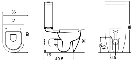
ART. 28013 vaso monoblocco BTW monobloc wc
